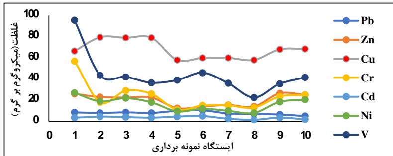
نمودار ۳- میانگین غلظت فلزات سنگین ( میکروگرم برگرم) در رسوبات متعلق به ایستگاه‌های مختلف
