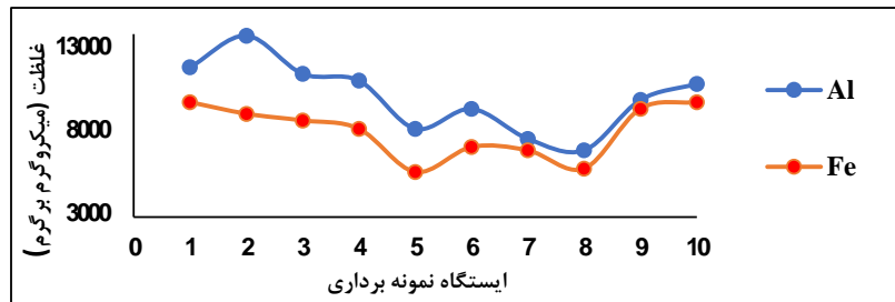
نمودار ۴- میانگین غلظت فلزات آهن و آلومینیوم ( میکروگرم برگرم) در رسوبات متعلق به ایستگاه‌های مختلف
