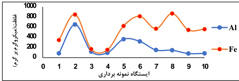
نمودار ۲- میانگین غلظت فلزات آهن و آلومینیوم ( میکروگرم برگرم) در صدف‌های متعلق به ایستگاه‌های مختلف
