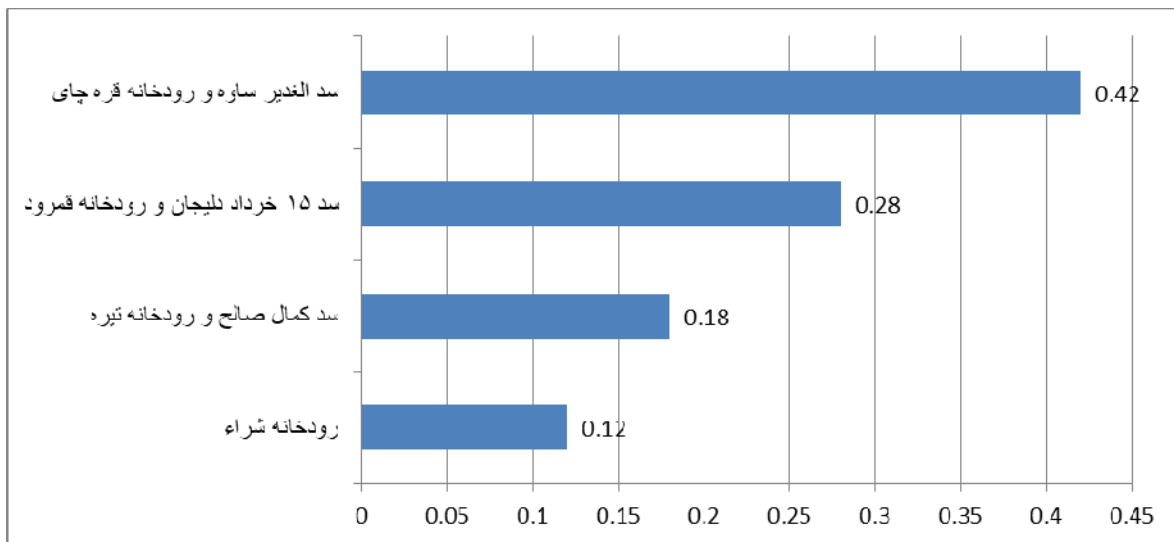
شکل ۶- نتایج ارزیابی کیفیت زیستگاه سنگ ( Lutra lutra ) در استان مرکزی با روش ANP
