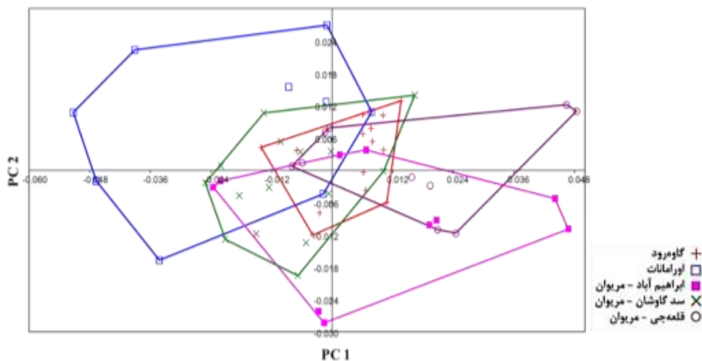
شکل ۳- تحلیل مولفه‌های اصلی (PCA) شکل بدن جمعیت‌های مورد مطالعه سیاه‌ماهی باله بلند.
