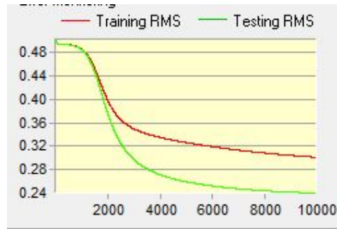
شکل ۳- نمودار خطای مربوط به مراحل آموزش و آزمون در فصول پاییز (سمت راست) و زمستان (سمت چپ)
